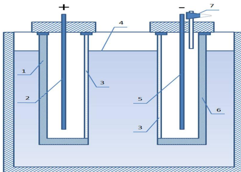
Рис. 1. Устройство для электрофизической активации: 1 – анодная камера, 2 – медный электрод, 3 – мембрана (фильтровальная ткань), 4 – уровень воды, 5 – электрод из нержавеющей стали, 6 – катодная камера, 7 – краник для катодного газа.
