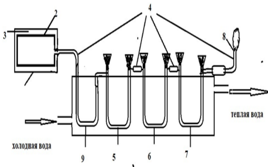
Сүрөт 1. Көмүрдү кокстоо процессин изилдөө үчүн орнотуу схемасы.
