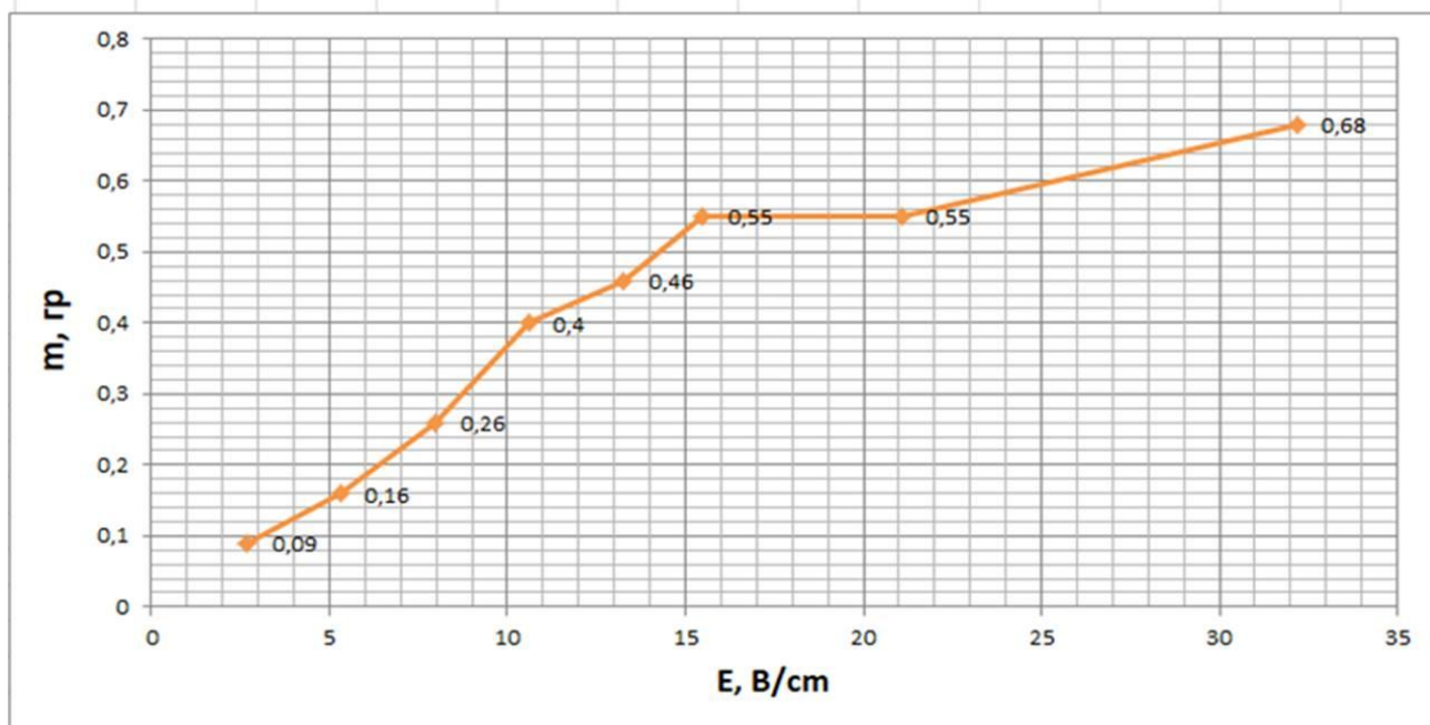
Рис. 3. График зависимости массы осадка в анодном электроде от напряженности электрического поля между электродами.
